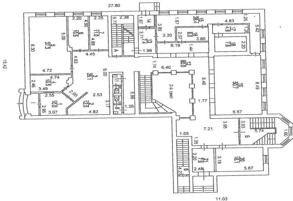
План 1 этажа
